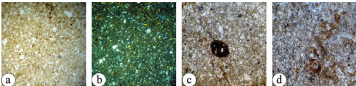
Рис. 11. Малий Раковець IV. Мікробудова удайського матеріалу (шурф №16): а – співрозмірність лесових часточок і зерен первинних мінералів; b – пилувато-плазмова мікробудова; c – залізисто-мангановий мікроорштейн; d – гумусово-глинисті і глинисті натеки в плазмі і навколо зерен скелету (a, c, d – нік. ||, b – нік. +, збільшення 100).
