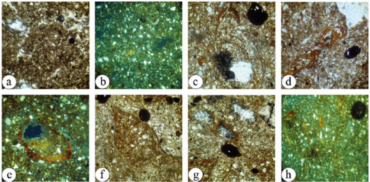
Рис. 12. Малий Раковець IV. Мікробудова витачівських ґрунтів (шурф №19):
