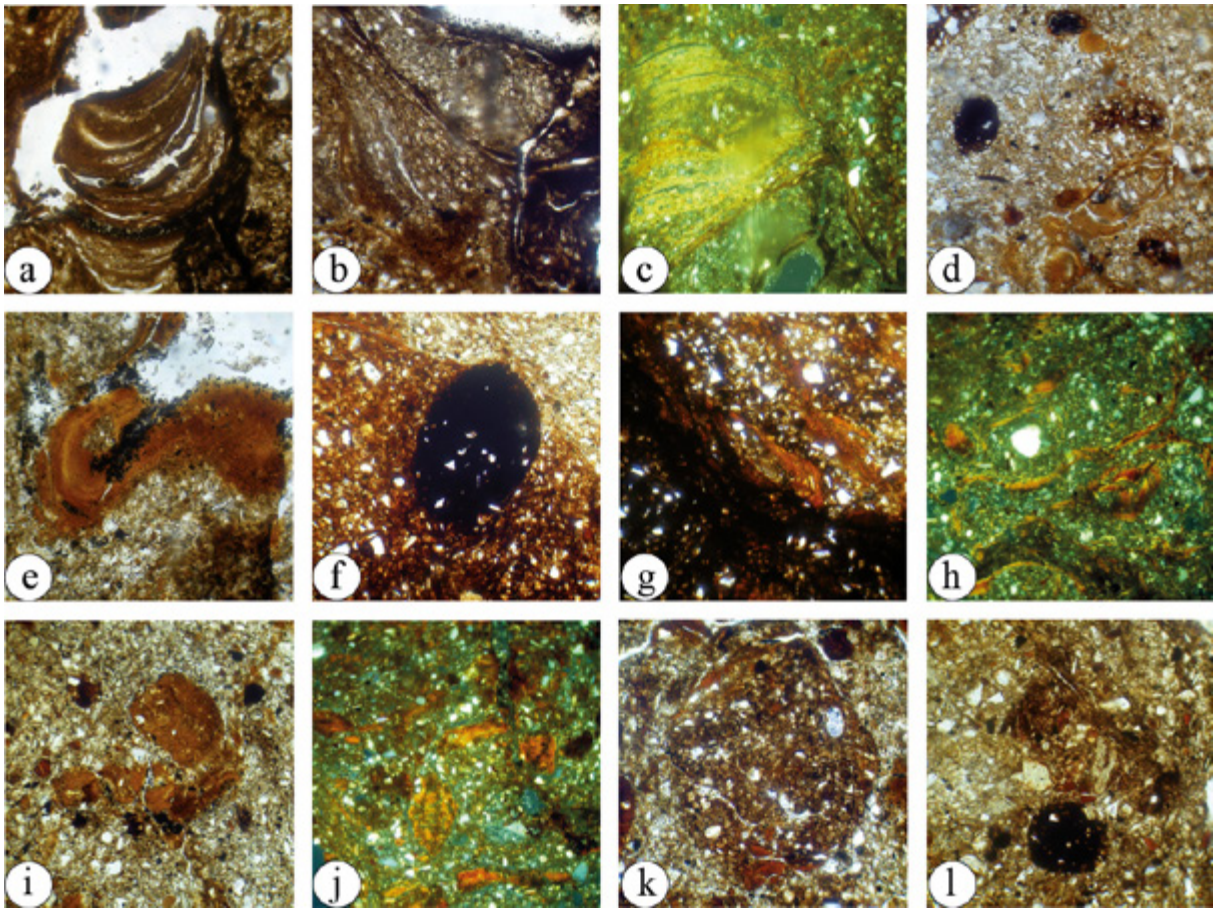
Рис. 10. Малий Раковець IV. Мікробудова прилуцького ґрунту (шурф №18):
