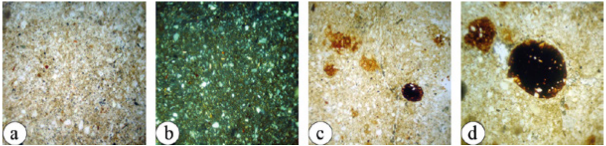
Рис. 8. Малий Раковець IV. Мікробудова дніпровського матеріалу (шурф №15): а – глинисті лесові часточки, співрозмірні із зернами первинних мінералів; б – пилувато-плазмова мікробудова; с – залізисті і манганові мікроорштейни і плями; d – крупні манганово-залізисті мікроорштейни (а, с, d – нік. ||, б – нік. +, збільшення 100).
