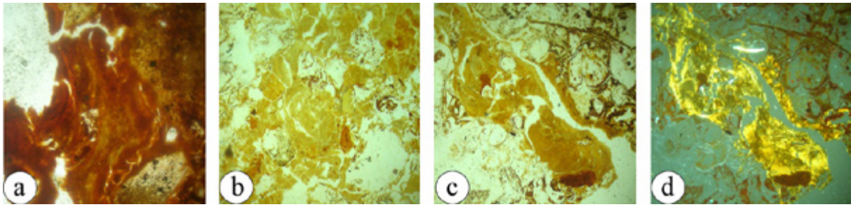
Рис. 6. Малий Раковець IV. Мікробудова мартоношського ґрунту (шурф №19): а – залізи́сто-глини́сті натеки; б, с, d – глини́сті і залізи́сто-глини́сті кутани ілювіювання (а – с – нік. ||; d – нік. +; збільшення 100).
