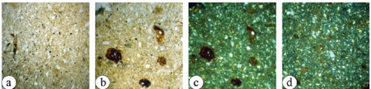
Рис. 13. Малий Раковець IV. Мікробудова бузького матеріалу (шурф №18): а, б, с – лесова мікробудова (лесові часточки, співрозмірні із зернами скелету), залізо-манганові мікроорштейни і плями; d – пилувато-плазмова мікробудова (а, б – нік. ||, с, d – нік. +, збільшення 100).
