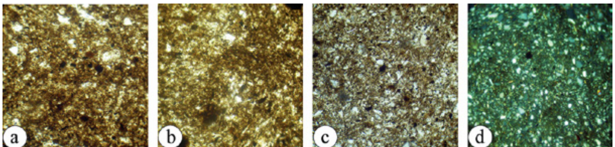
Рис. 14. Малий Раковець IV. Мікробудова голоценового ґрунту (шурф №19): а, б – складні мікроагрегати II порядку, розділені порами; с – рівномірне просочення плазми органо-глинистою речовиною; d – пилувато-плазмова мікробудова (а – с – нік. ||, d – нік. +, збільшення 100).
