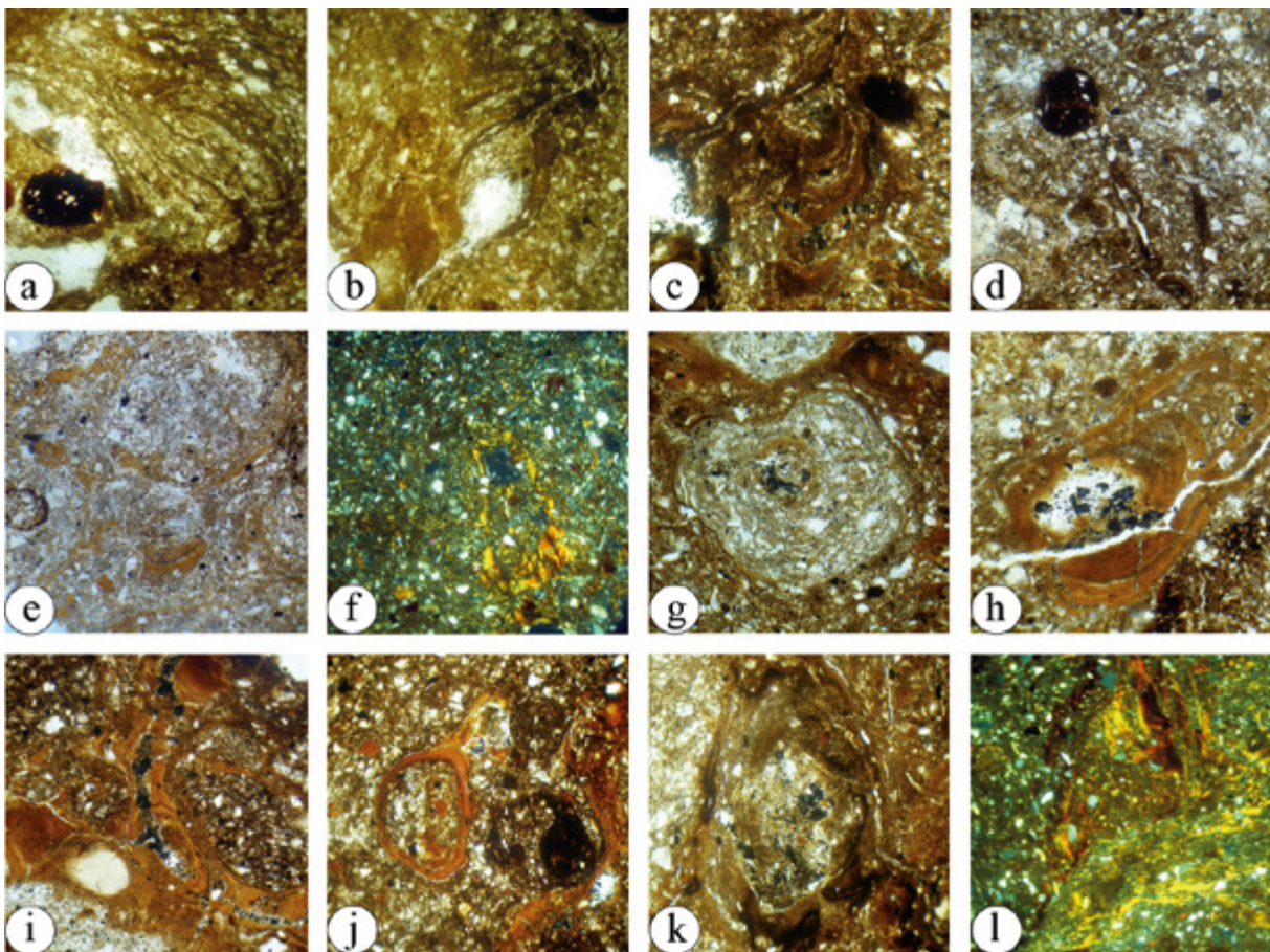
Рис. 7. Малий Раковець IV. Мікробудова завадівського (zv3) ґрунту (шурф №15): а – гумусово-глини́сті натеки навколо зерен скелету, залізи́сто-мангановий мікроорштейн; б – глини́сті і гумусово-глини́сті кутани; с – глини́сті і залізи́сто-глини́сті натеки з включенням часточок гумусу і зерен скелету, залізи́сто-мангановий мікроорштейн; d – залізи́сто-мангановий мікроорштейн і гумусово-глини́сті кутани навколо зерен скелету; e – глини́сті кутани; f – пилувато-плазмова мікробудова, залізи́сто-глини́сті кутани; g – гумусові і гумусово-глини́сті кутани (з включенням зерен скелету) з коломорфними залізи́сто-глини́стими плівками; h – залізи́сто-глини́сті натеки коломорфних глин навколо пори з включенням грубих часточок гумусу і зерен скелету; i – концентрація залізи́сто-глини́стої речовини біля зерен скелету, пори заповнені скелетанами з гумусово-глини́стими натеками; j – округлі скупчення органічно-глини́стої і залізи́сто-глини́стої речовини та залізи́сто-глини́сті і глини́сті натеки в плазмі, залізи́сто-мангановий мікроорштейн; k – гумусово-глини́сті і глини́сті кутани ілювіювання в плазмі з включенням оксидів і гідроксидів заліза і мангану; l – залізи́сто-глини́сті натеки коломорфних глин (a – e, g – k – нік. ||, f, l – нік. +, збільшення 100).
